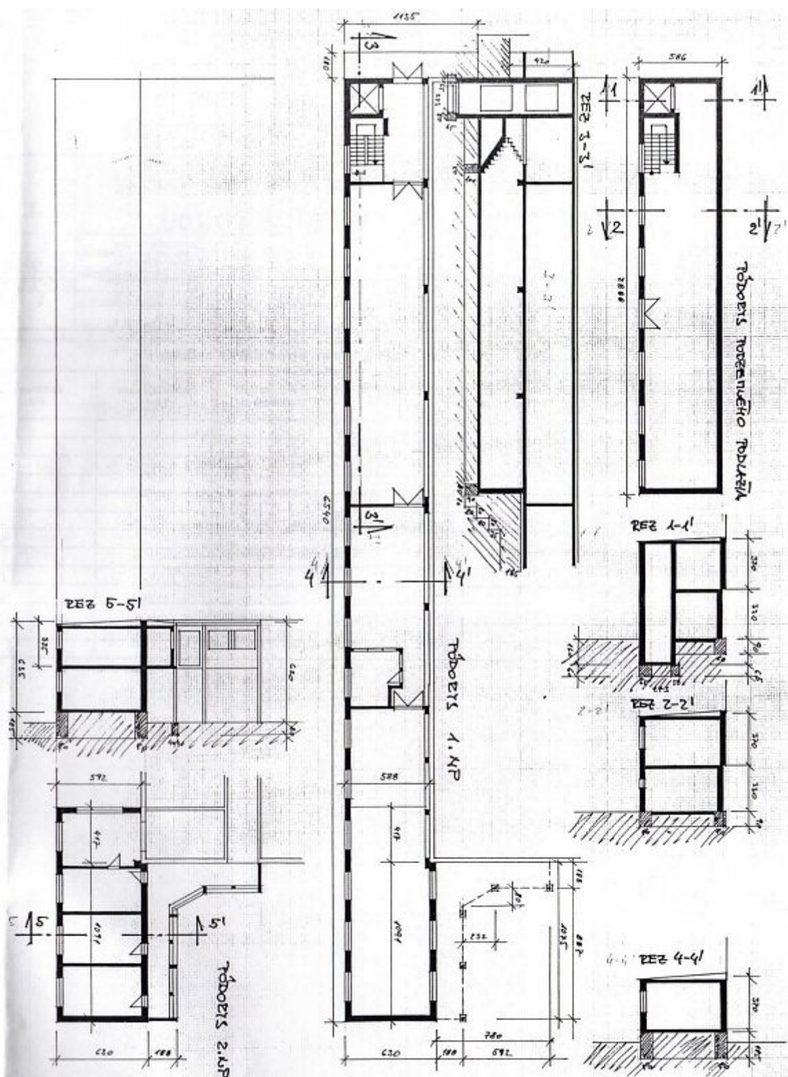
PRÍSTAUBA PREVÁDZKOVEJ BUDOVY ORIENTAČNÉ PÓDORYSY A REZY
